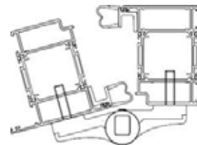
Klämskydd
